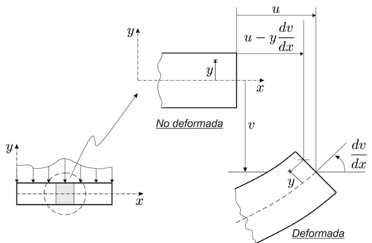
Figura 5. Cinemática de la viga de Euler-Bernoulli. Elaboración: Jaime Retama Velasco.
